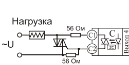
Подключение внешнего симистора
